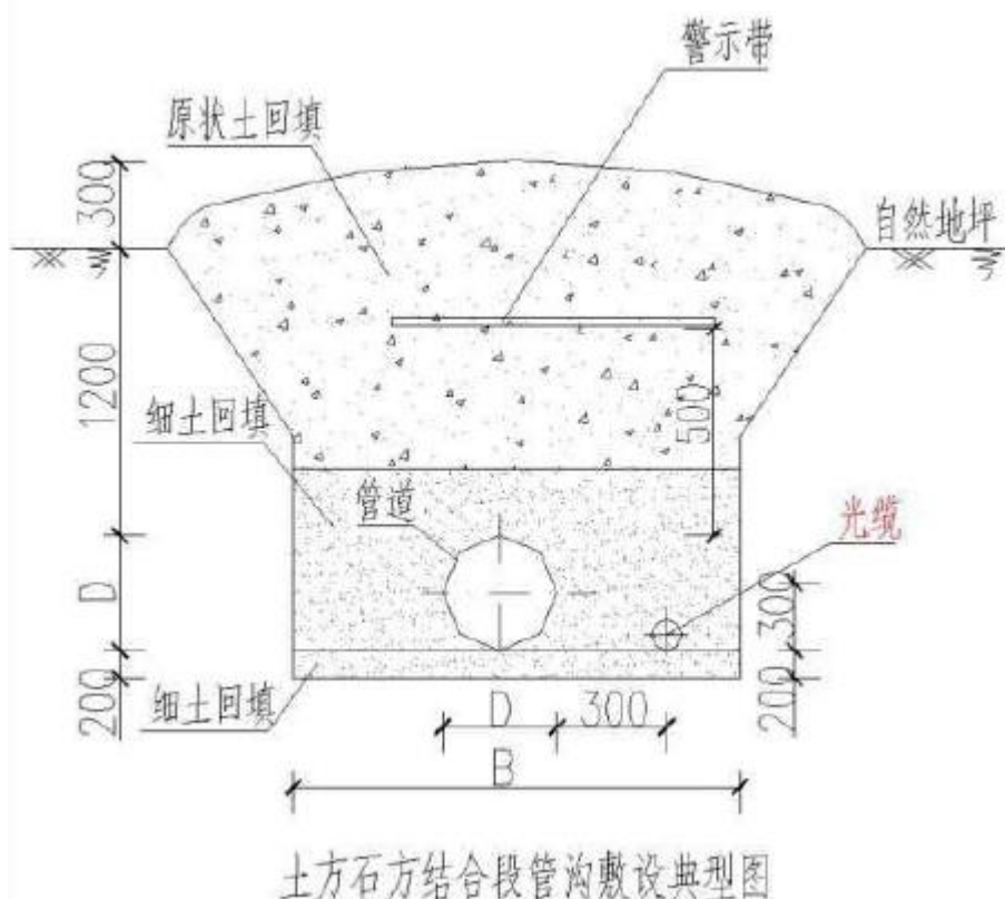
图 3.3-8 土石方结合段管沟敷设典型图
